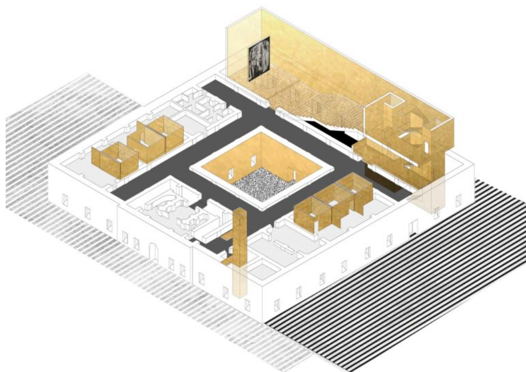
ESPLOSO ASSONOMETRICO
